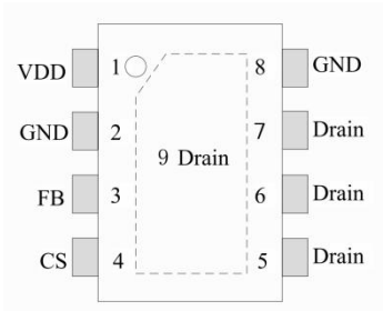
ESOP-8 俯视图
